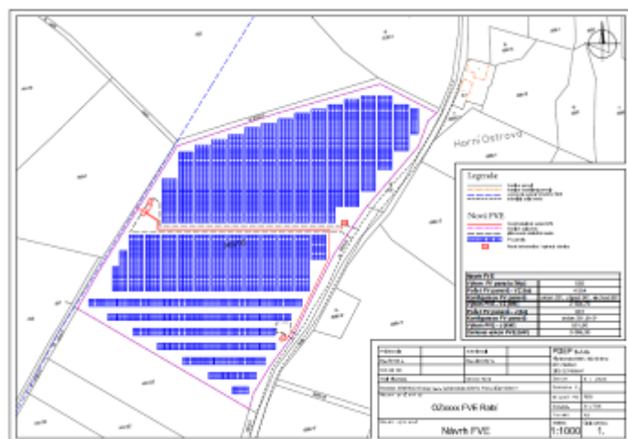
Plánované rozmístění FVE Rabí. Zdroj: ZENERGO Energy
